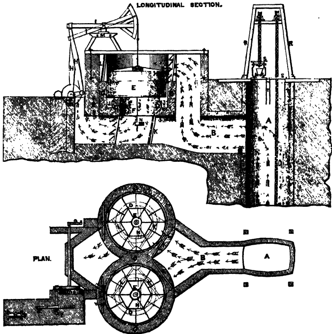
Fig. 46. Struve's Apparatus.
